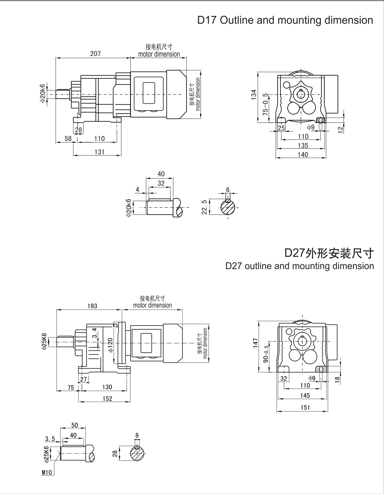
D17外形安装尺寸 D17 outline and mounting dimension
